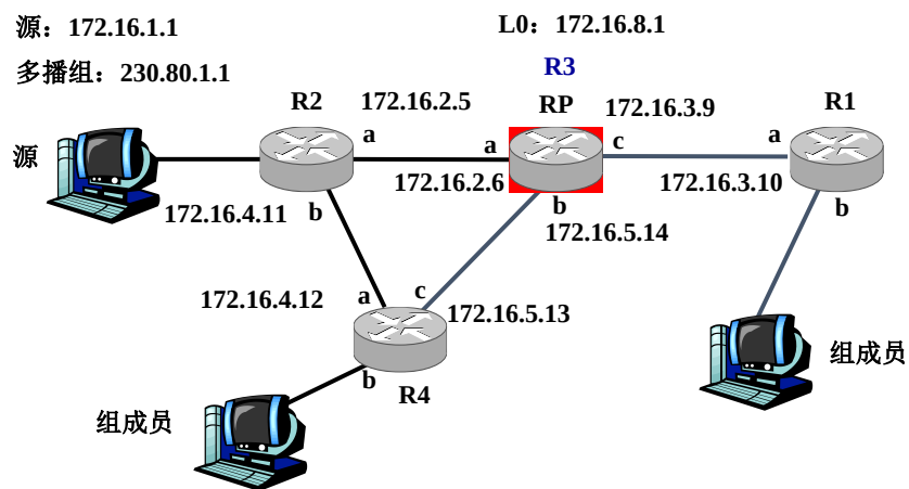
多播源到 RP 对应的基于源的树多播表（16 分）
